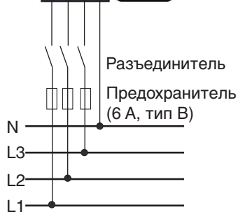
Рис. Пример подключения: измерение напряжения через разъединитель и предохранители.
