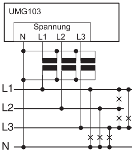
Рис. Пример подключения для измерения напряжения через трансформатор напряжения.
