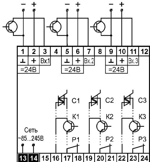
Схема подключения
