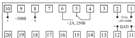
Рис. 8 – Клеммник P94-V-1-0.5-K-I420-ACX220
