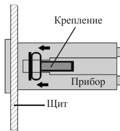
Рис. 3 – Установка прибора
