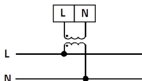
Рис. 3 – Подключение через трансформатор напряжения (если напряжение > 600\text{В} )
