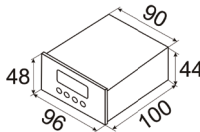
Рис. 9 – Размеры. Тип корпуса P94
