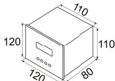
Рис. 11 – Размеры. Тип корпуса P1212
