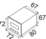
Рис. 8 – Размеры. Тип корпуса P77
