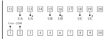
Рис. 9 – Клеммы подключения. Тип корпуса P99
