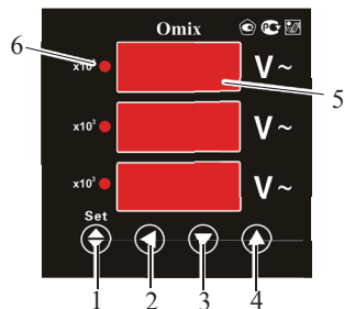
Рис. 1 – Управляющие элементы
