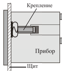
Рис. 2 – Установка прибора
