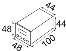
Рис. 13 – Размеры. Тип корпуса P44
