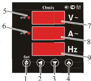
Рис. 1 – Управляющие элементы
